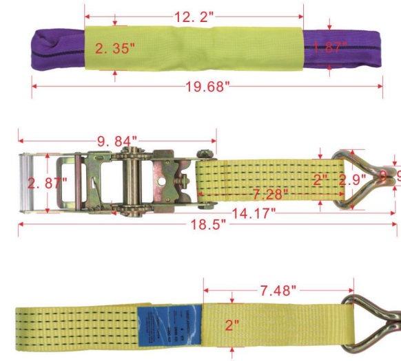
型号 (Item No): XQK-012
