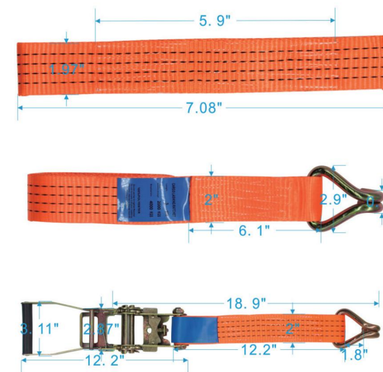
型号 (Item No): XQK-010
